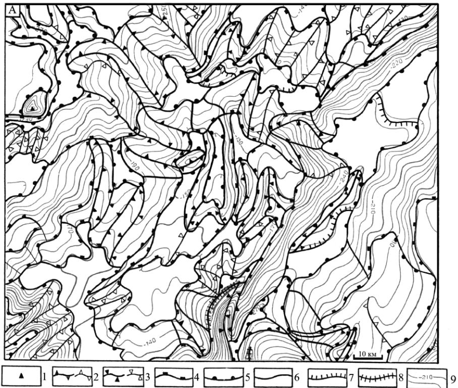
Рис. 16. Примеры предварительных геоморфологических карт: А – выполненной по упрощенной схеме, Б – выполненной по полной схеме с использованием векторных линий.
