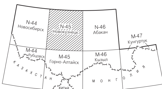
Схема расположения листов Алтае-Саянской серии
