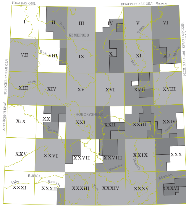
СХЕМА ИСПОЛЬЗОВАННЫХ МАТЕРИАЛОВ Масштаб 1 : 5 000 000
