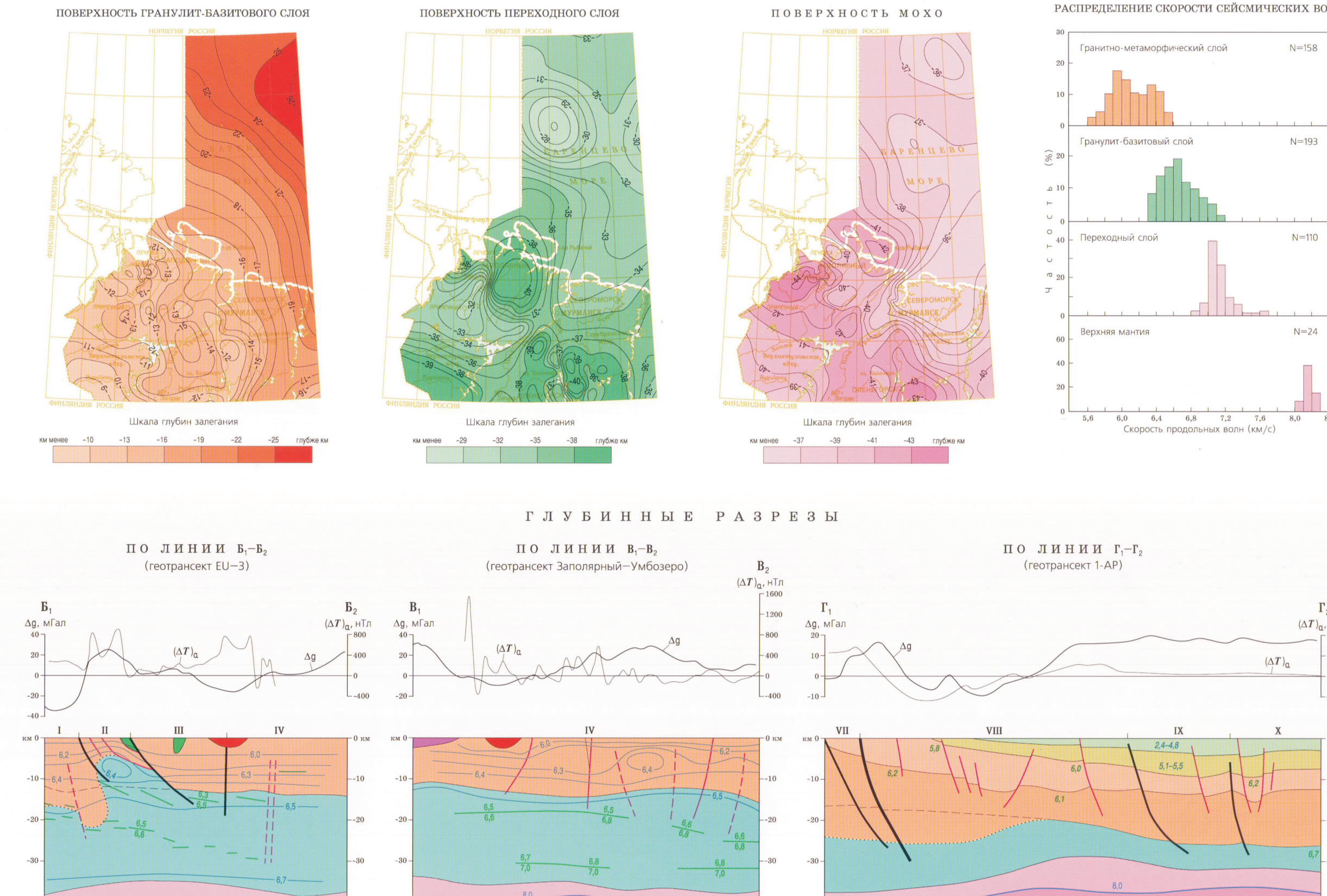
СХЕМЫ ГЛУБИНЫ ЗАЛЕГАНИЯ ГРАНИЦ ЗЕМНОЙ КОРЫ. Масштаб 1 : 5 000 000
