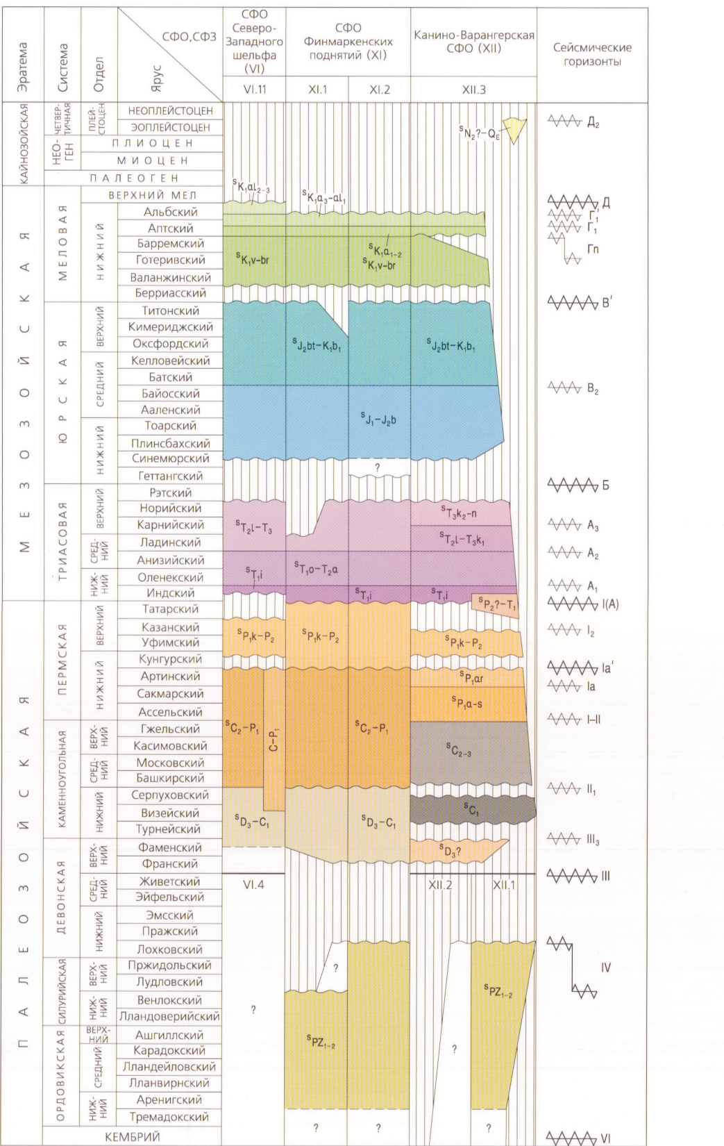
СХЕМА КОРРЕЛЯЦИИ КАРТОГРАФИРУЕМЫХ ПОДРАЗДЕЛЕНИЙ ПАЛЕОЗОЯ-КАЙНОЗОЯ БАРЕНЦЕВОМОРСКИЙ БЛОК
