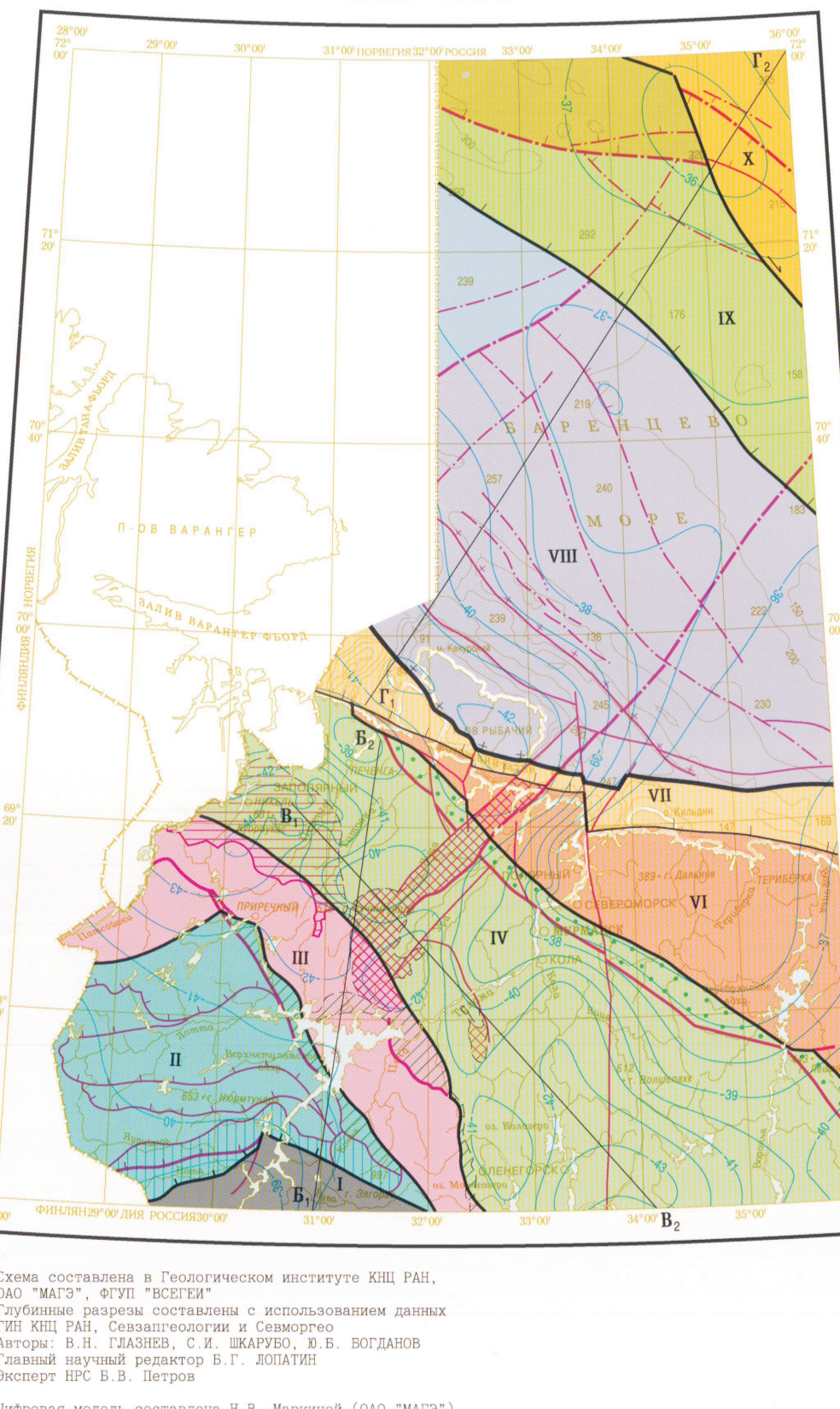
СХЕМА ГЛУБИННОГО СТРОЕНИЯ ЗЕМНОЙ КОРЫ Масштаб 1 : 2 500 000
