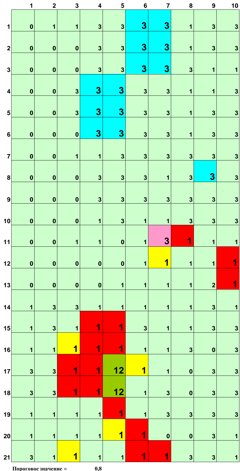
Рис.4.3.1 Прогнозная схема, построенная с помощью программы ПРОТЕЙ-6 Бледно-зеленым цветом показаны неперспективные участки, красным - участки с известными золоторудными месторождениями, желтым - перспективные участки с предполагаемым внутрирудным уровнем эрозионного среза рудных объектов, голубым - с дальним надрудным, травяным - с внутрирудным и ближним надрудным, сиреневым - дальним надрудным в пределах участков с известными месторождениями.
