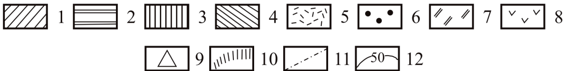
Рис. 5.4.1. Карта кор выветривания правобережья р. Подкаменная Тунгуска. Составили В. С. Певзнер, И. И. Кунгурцев, 1972 г.
