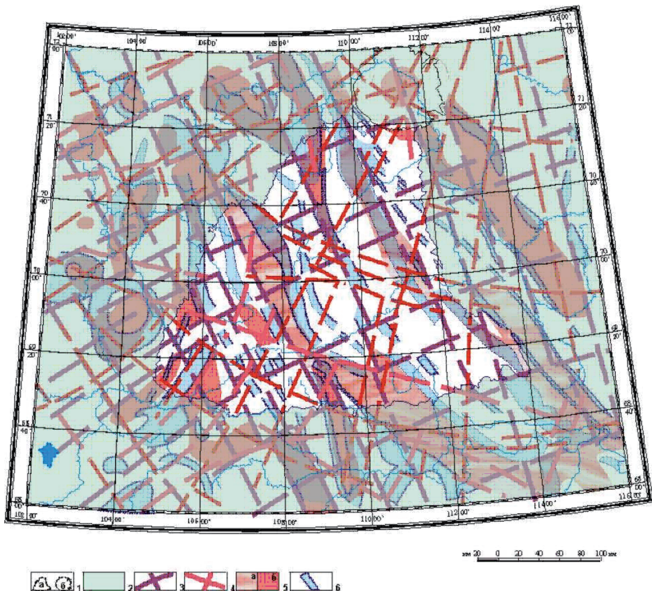
Рис. 6.2.6. Специализированная на золото (золото-кварцевая формация) геолого-структурная карта Анабарского щита.
