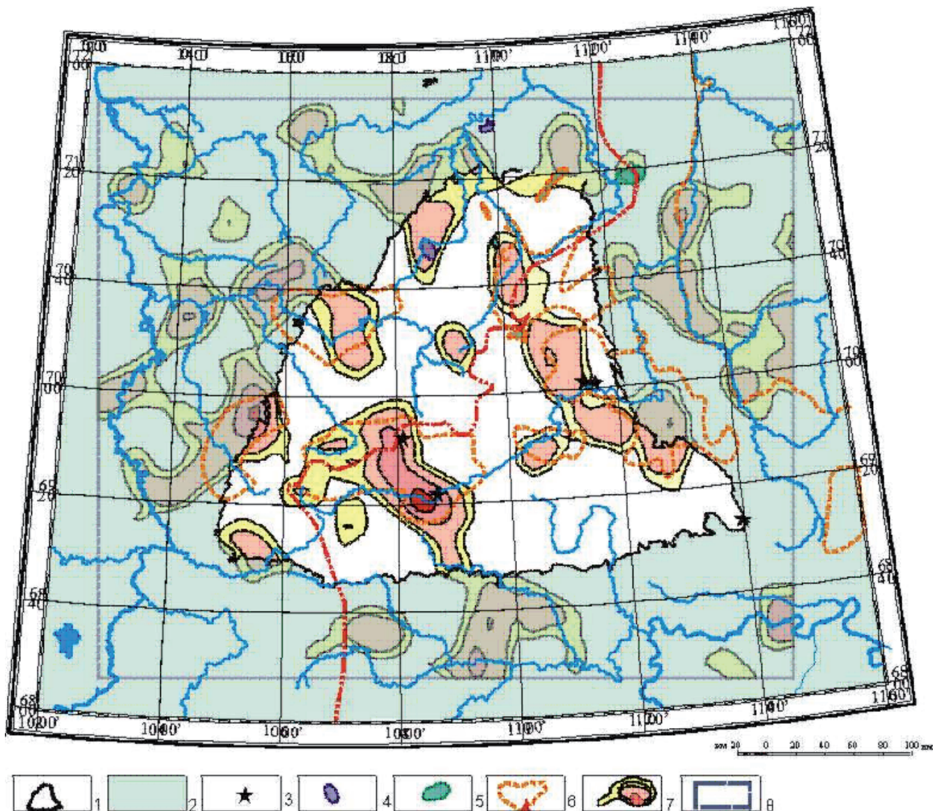
Рис. 6.2.7. Схема размещения участков, благоприятных по комплексу дистанционных признаков для локализации оруденения золото-кварцевой формации в фундаментах древних платформ.
