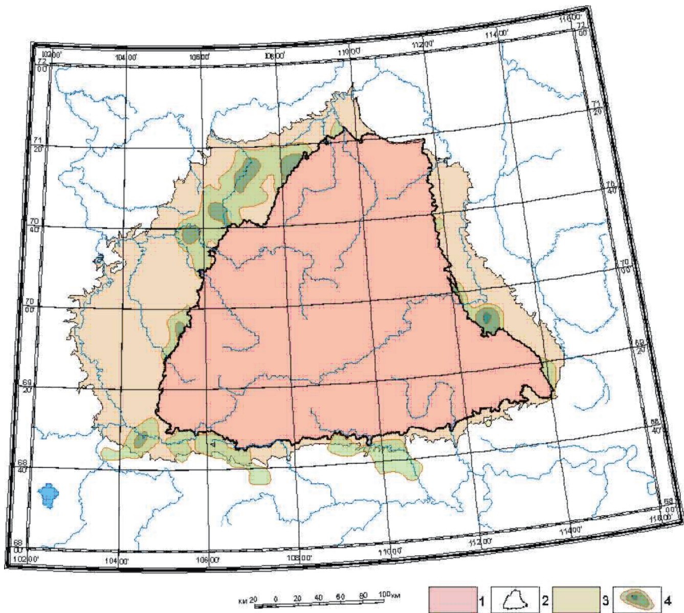
Рис.6.2.8. Схема участков, благоприятных для формирования урановых месторождений в связи с зонами «несогласия».
