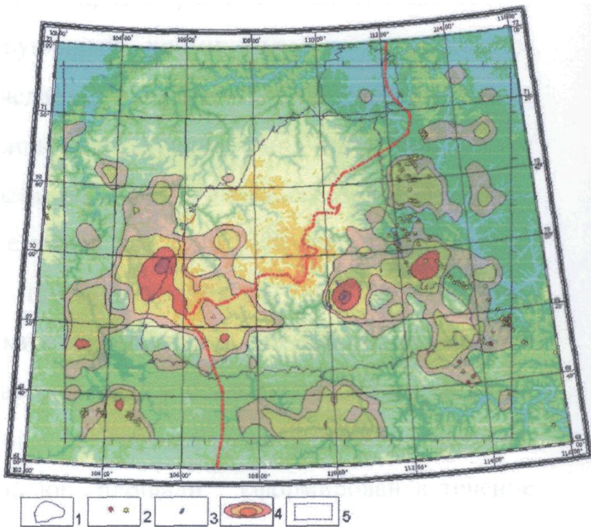
Рис. 6.2.9. Схема участков, благоприятных (по сумме структурных факторов) для локализации кимберлитов.
