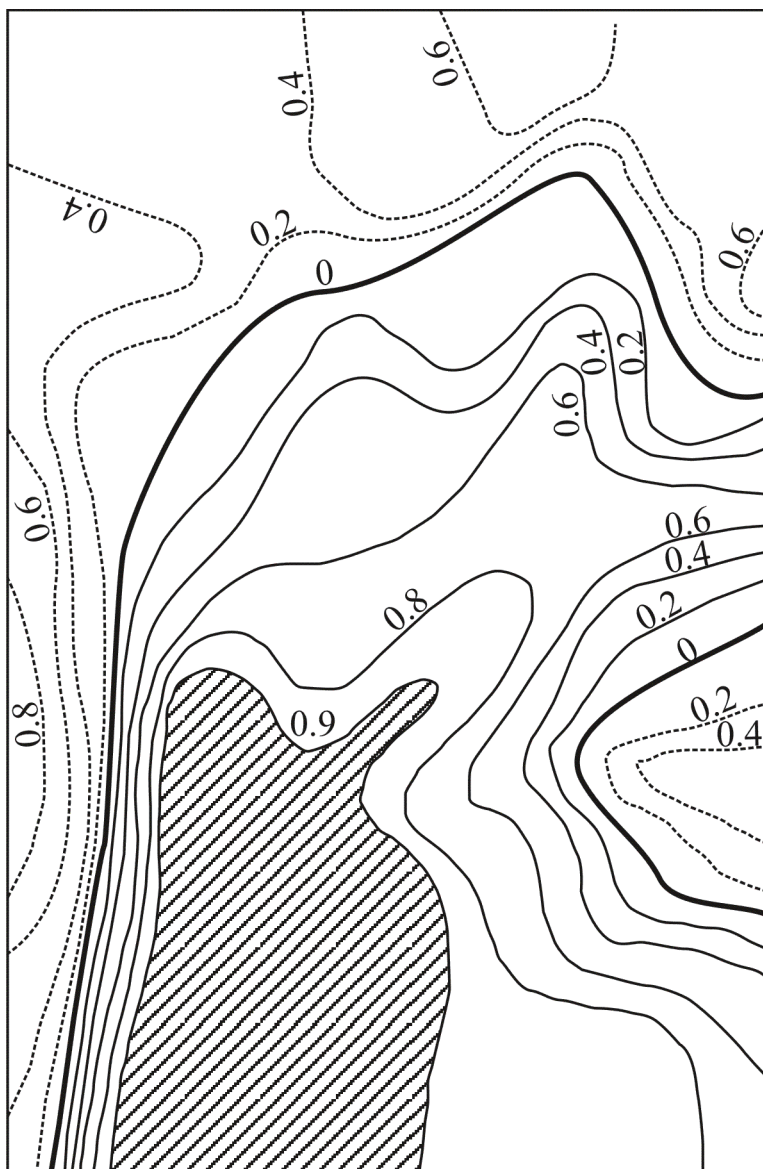
Рис. 6.4.1 — Карта изокоррелят никель-кобальт в районе погребенной залежи силикатного никеля.
