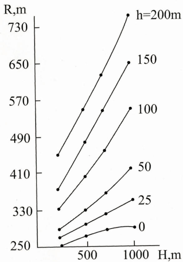
Рис.7.2. Зависимость расстояния R (см.рис.7.1) от вертикальной мощности цилиндра H для различных мощностей немагнитного покрова h (по Г.Б.Романовскому)
