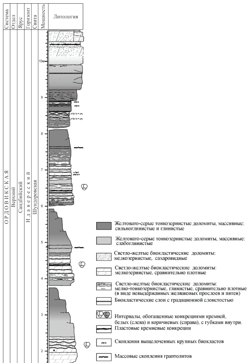
Разрез шундоровской свиты в карьере Каськово
