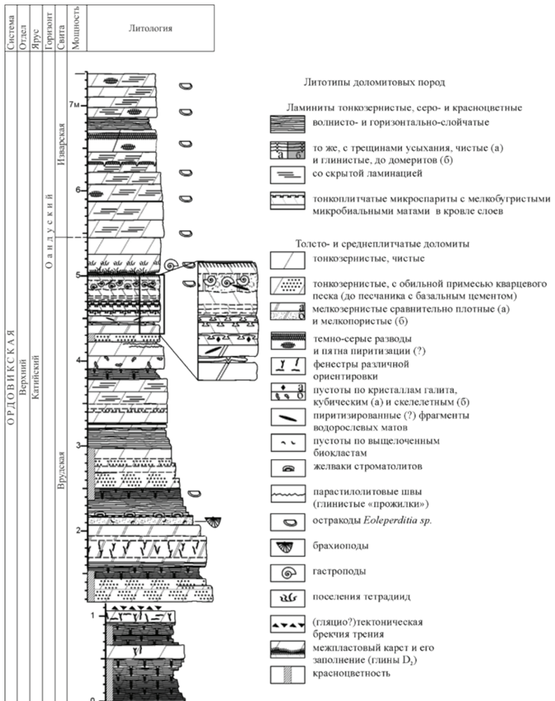
Разрез врудской и изварской свит в карьере Волосово
