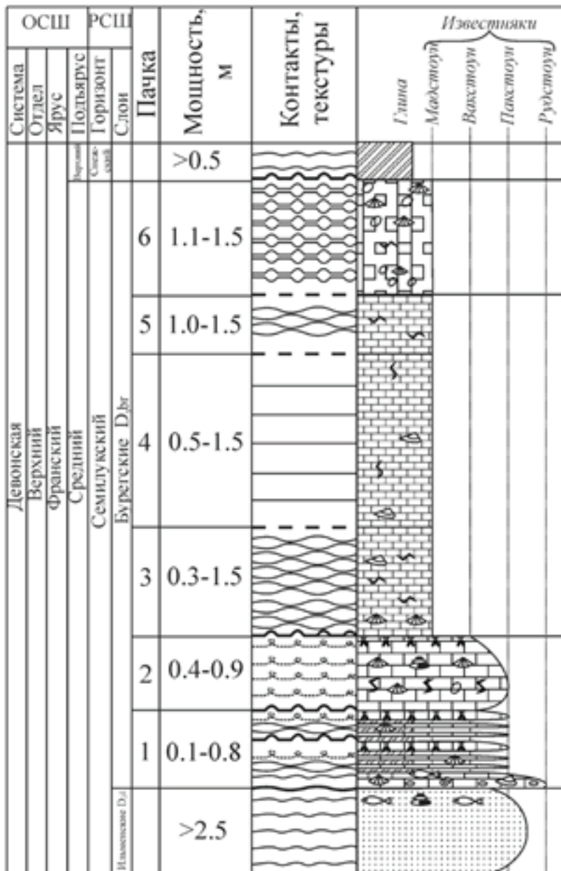
Разрез «Буреги», стратотип бургеских слоев (Русецкая и др., 2013)
