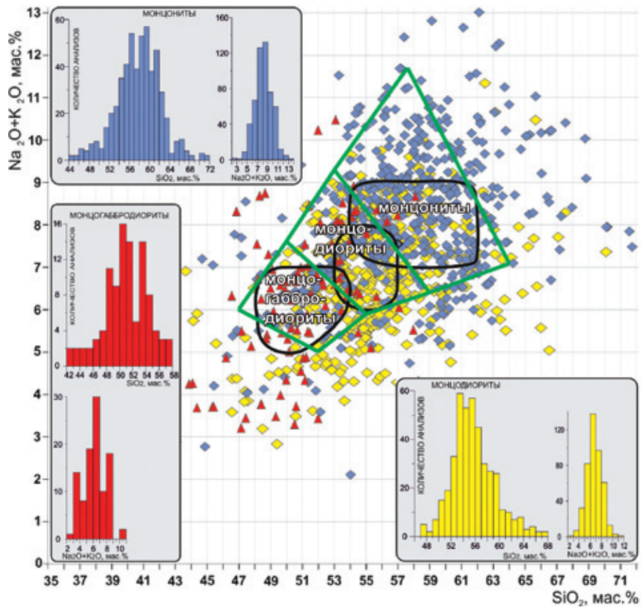
Рис. 4. Области максимальной концентрации химических параметров (на основе гистограмм) и границы полей монцогаббродиоритов – монцодиоритов – монцитонитов на диаграмме \Sigma\text{Alk} - \text{SiO}_2
