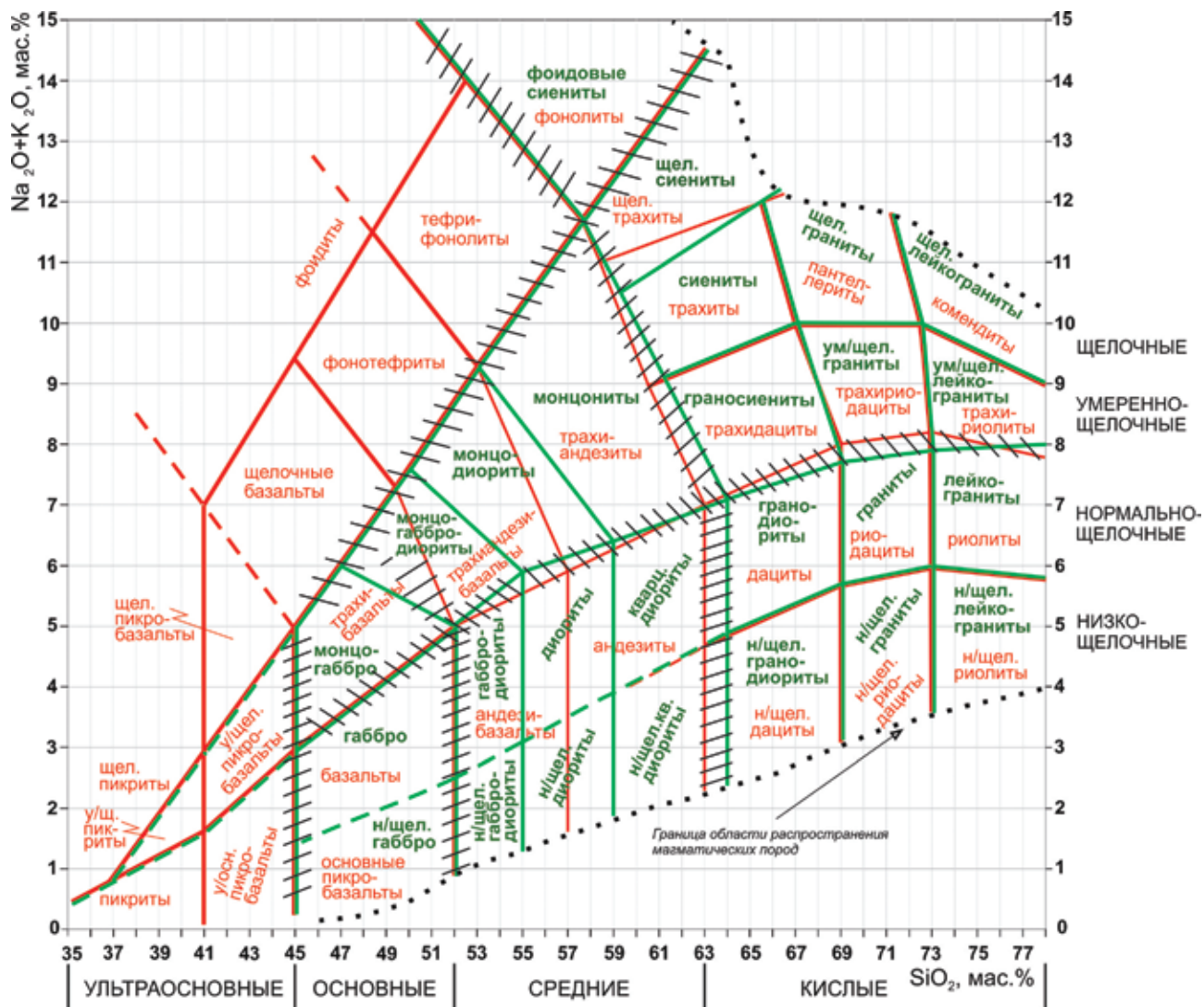
Рис. 9. Границы полей групп plutonic (зеленые линии) и вулканических (красные линии) горных пород на TAS-диаграмме. Заштрихованы основные пограничные «зоны неопределенности» между группами пород
