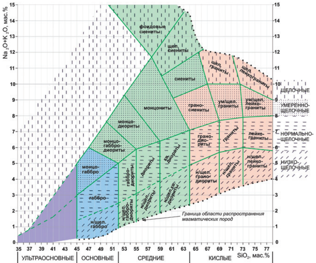
Рис. 8. Диаграмма сумма щелочей – кремнезем (TAS) для химической классификации плутонических горных пород основного, среднего и кислого составов
