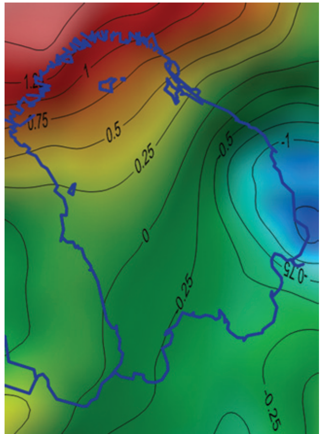
Рис. 9. Приблизительные оценочные ундуляции эквипотенциальной поверхности на примере геоида EGM2008 [33] относительно условной нулевой линии Кронштадта
