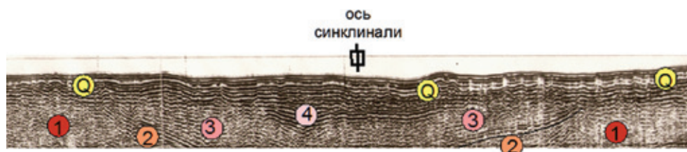
Рис. 4. Сейсмостратиграфическая выраженность Вуоксинской синклинали в западной части 1 – комплекс, отвечающий раннерифейским образованиям; 2–4 – более молодые подразделения, характеризуется отчетливым резким конседиментационным увеличением мощности. Q – четвертичные отложения
