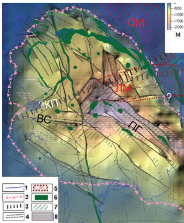
Рис. 3. Схема тектонического содержания для рифейских этапов
