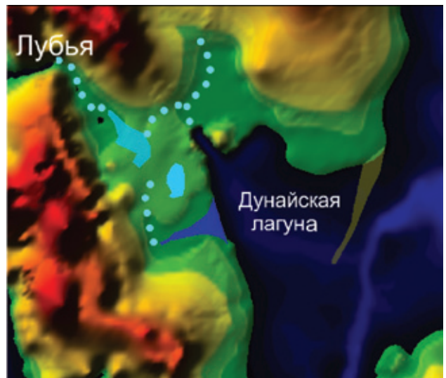
Рис. 10. Низина Лубья, разделяющая Колтушскую и Румболовско-Кяселевскую возвышенности как потенциальный элемент позднепоследнего Балтийско-Ладожского соединения
