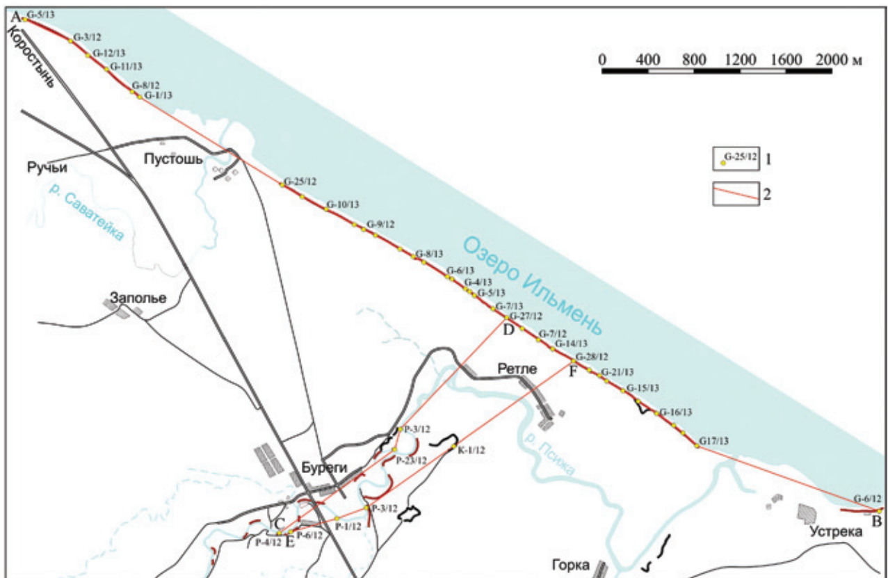
Рис. 1. Схема расположения изученных обнажений пачки ракушняковых известняков бурегских слоев и линий литологических разрезов в районе южного берега оз. Ильмень
