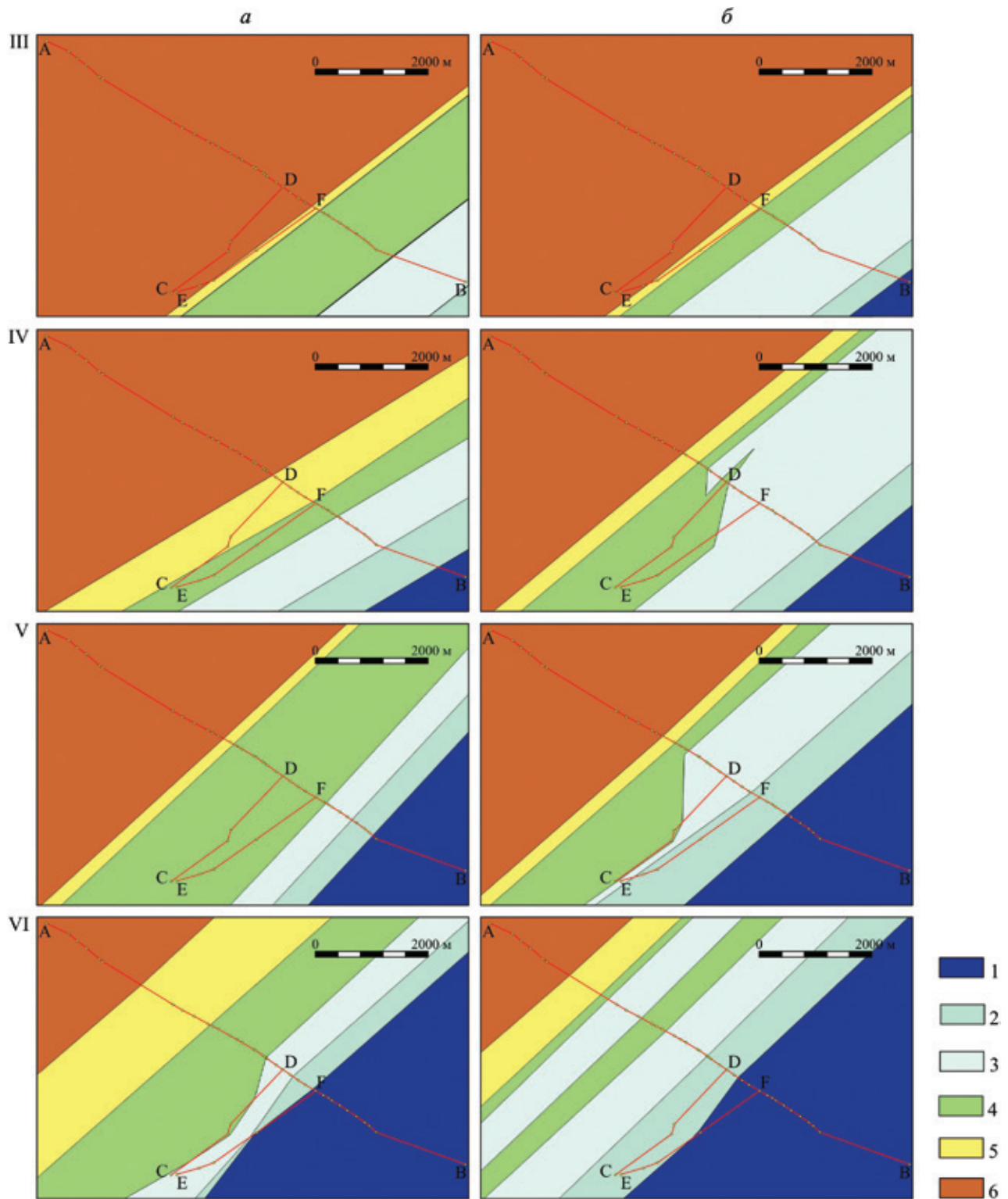
Рис. 5. Палеогеографические схемы для начальных (а) и финальных (б) стадий формирования III, IV, V и VI клиноформ пачки ракушняковых известняков
