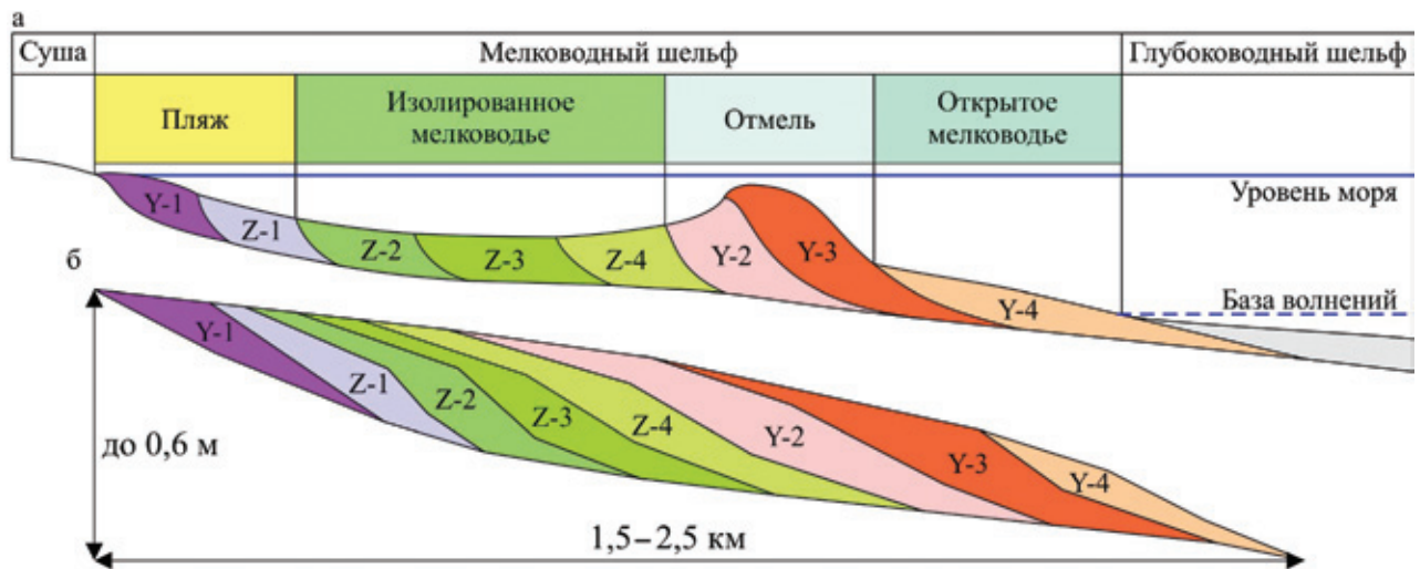
Рис. 3. Обстановки накопления пачки ракушняковых известняков (а) и схема строения клиноформы – геологического тела, формировавшегося в результате заверщенного трансгрессивного цикла их эволюции (б). Расшифровку буквенно-цифровых индексов см. в тексте
