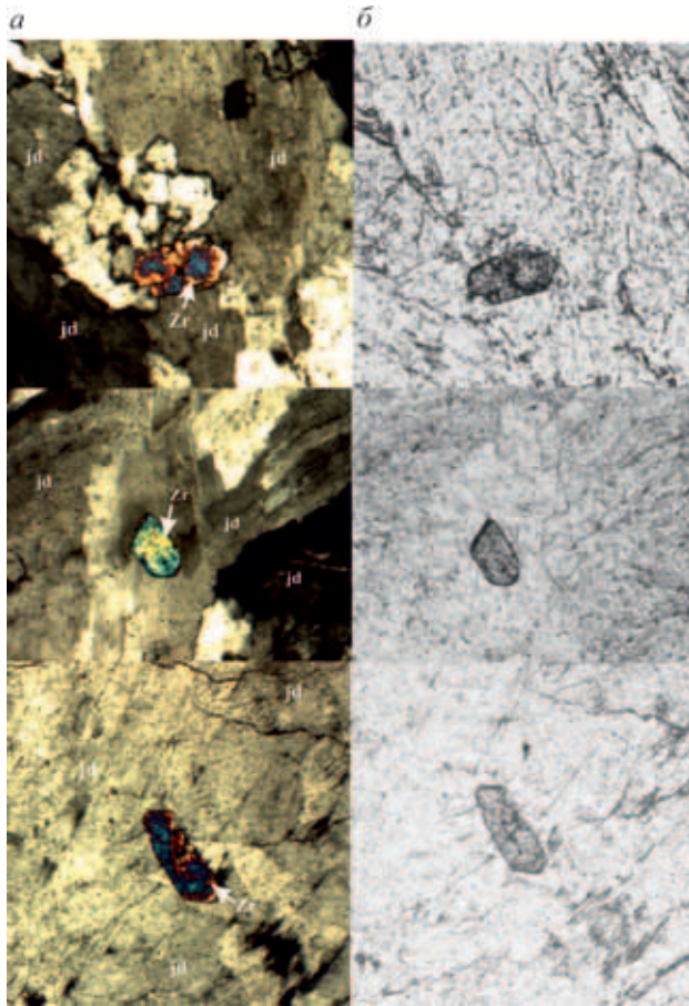
Рис. 2. Зерна цирконов в жадеитите ( \times 10 ), обр. 3537 a – в скрещенных николях, б – в проходящем свете
