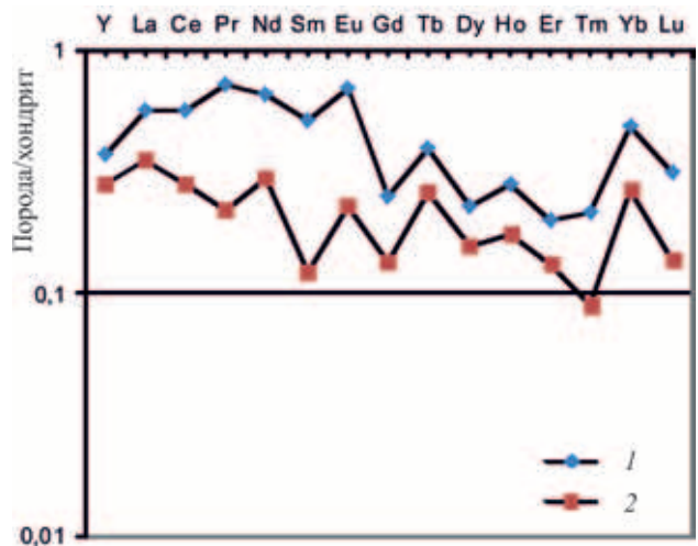
Рис. 3. Спайдер-диаграмма распределения редкоземельных элементов в жадеитите
