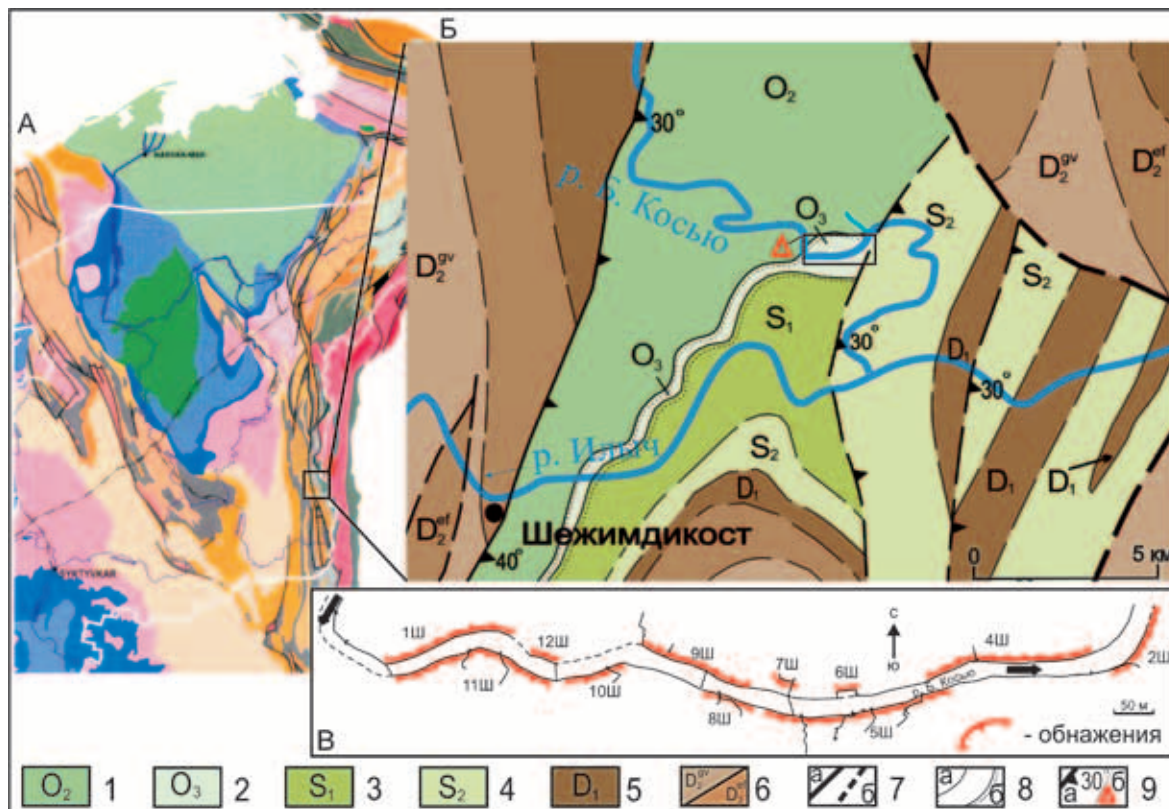
Рис. 1. Район исследований. А, Б – геологическая карта (по В. В. Юдину, 1983, с доп.); В – схема расположения выходов верхнеордовикских карбонатных отложений на р. Б. Косью
