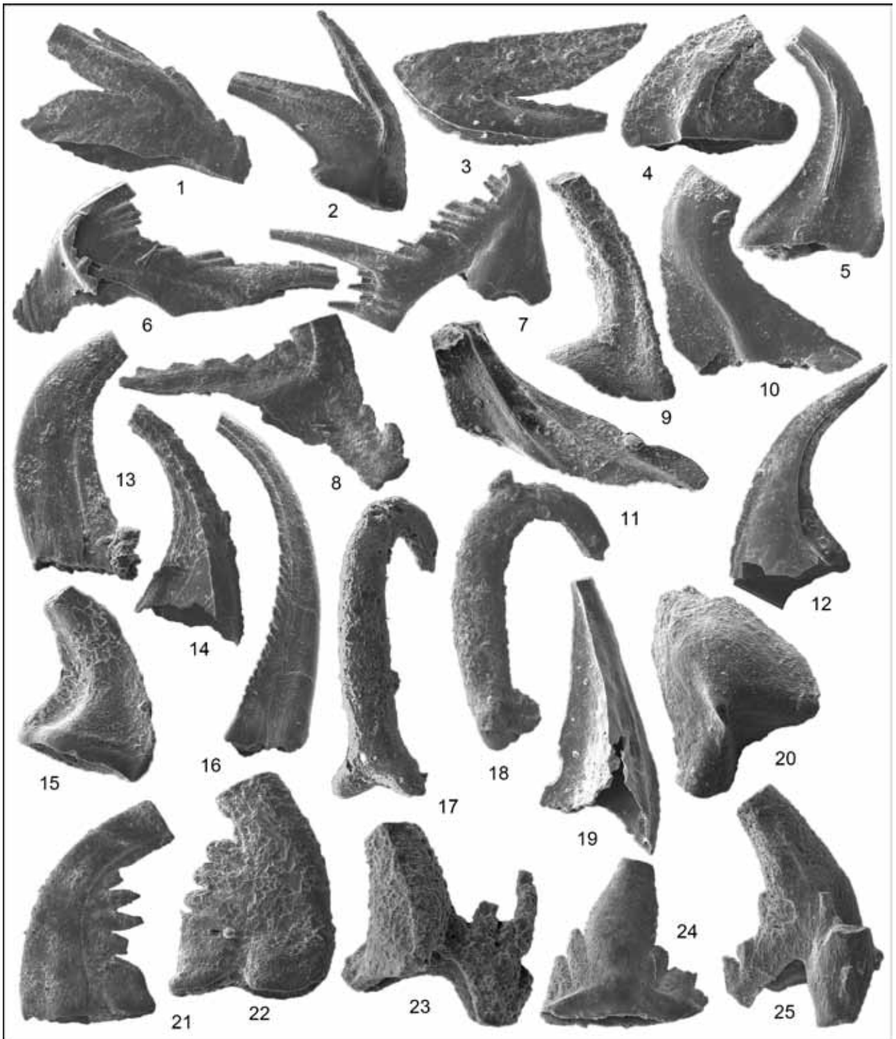
Рис. 3. Конодонты из разреза р. Б. Косью (Северный Урал)
